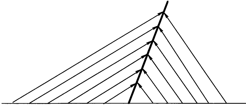
k -shock wave
