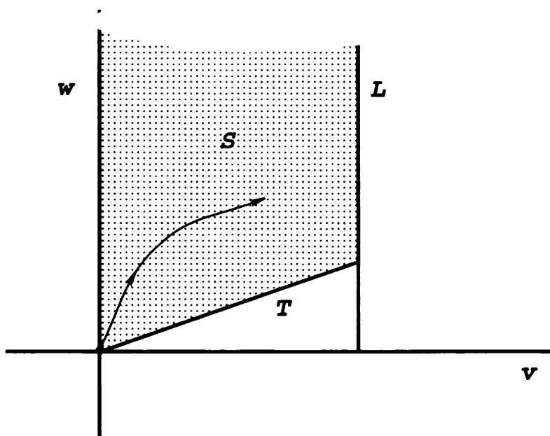
The region S
