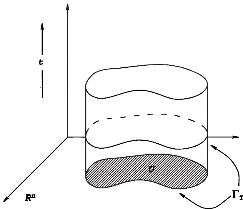
The region U_T
