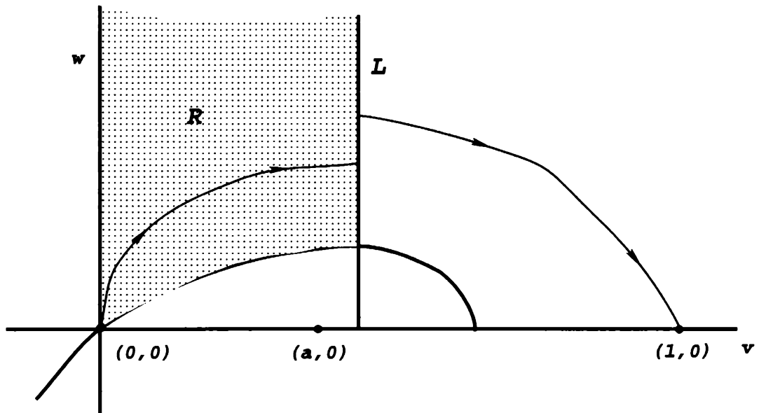
The region R
